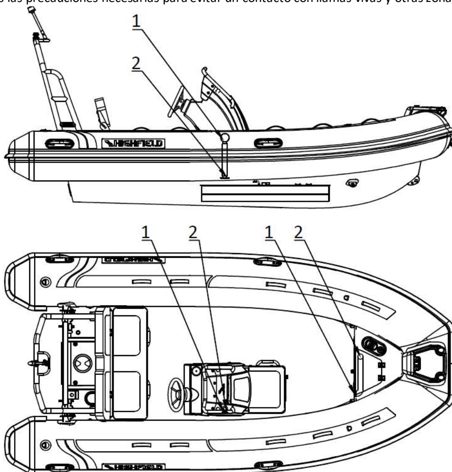
Diagrama del diseño de ventilación del compartimento del depósito de combustible (CL420-460)
