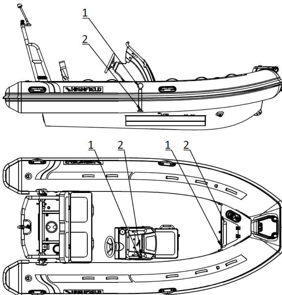
Darstellung der Tankraumbelüftung (CL420-460)
