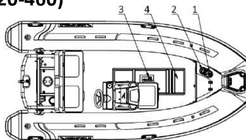
Darstellung Kraftstoffsystem
