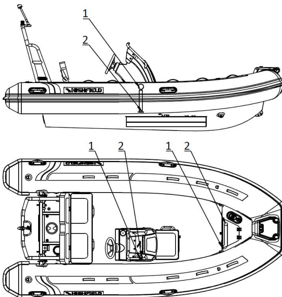
Schéma d'implantation de la ventilation du compartiment du réservoir d'essence. (CL420-460)
